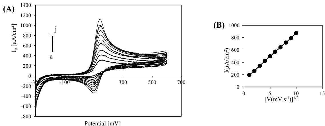
Fig.5 : (A) CVs of DA in pH 7.4 PBS at various scan rates: (a) 10\text{mVs}^{-1} ; (b) 20\text{mVs}^{-1} ; (c) 30\text{mVs}^{-1} ; (d) 40\text{mVs}^{-1} ; (e) 50\text{mVs}^{-1} ; (f) 60\text{mVs}^{-1} ; (g) 70\text{mVs}^{-1} ; (h) 80\text{mVs}^{-1} ; (i) 90\text{mVs}^{-1} ; (j) 100\text{mVs}^{-1} . (B) Plots of I_{pa} vs. Scan rates.
