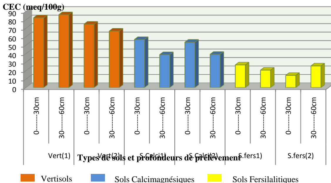
Figure 5 : Distribution des sols en fonction de leur teneur en CEC.
