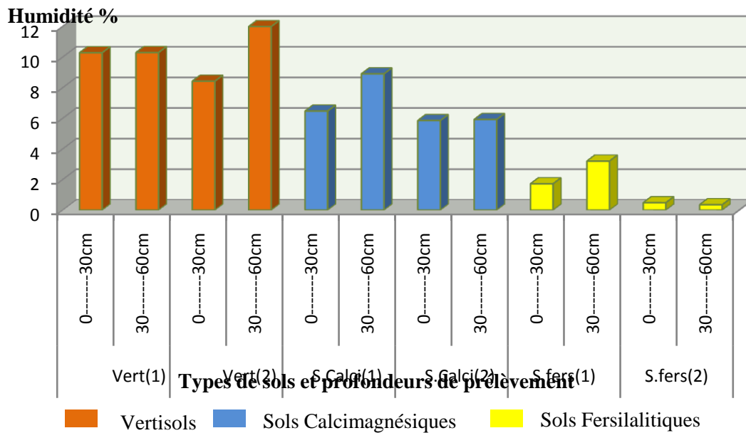
Figure 7 : Distribution des sols en fonction de leur pourcentage en humidité.
