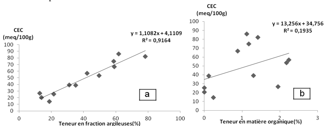
Figure 6 : Relations entre teneur en fraction argileuse et CEC (a) et entre teneur en matière organique et CEC (b).
